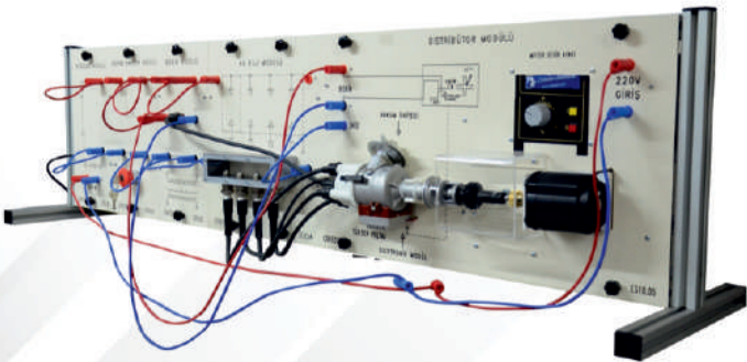
COK-ES10 Klasik Ateşleme Eğitim Seti
