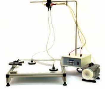
MK-503 Hava Masası Eğitim Seti
