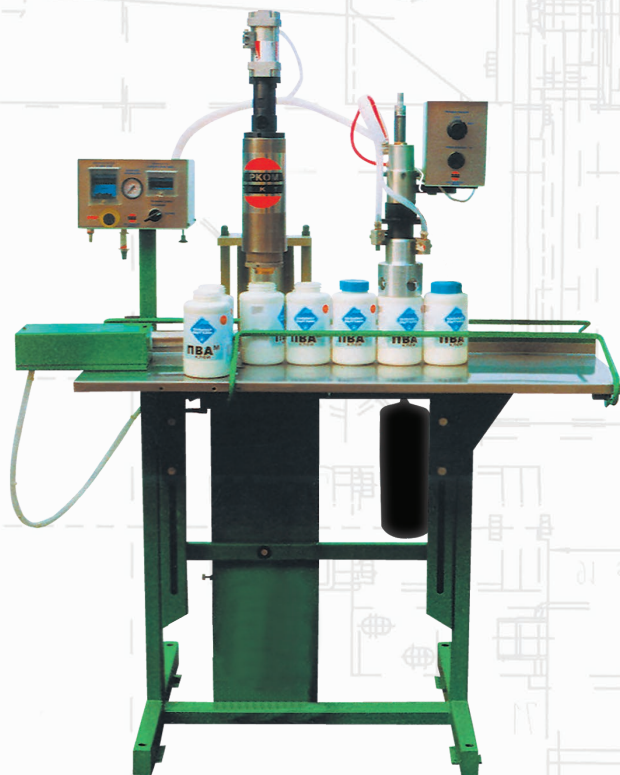
PRK.08B-SP.SN.1020.00 ПРК.08Б-СП.СН.1020.00
